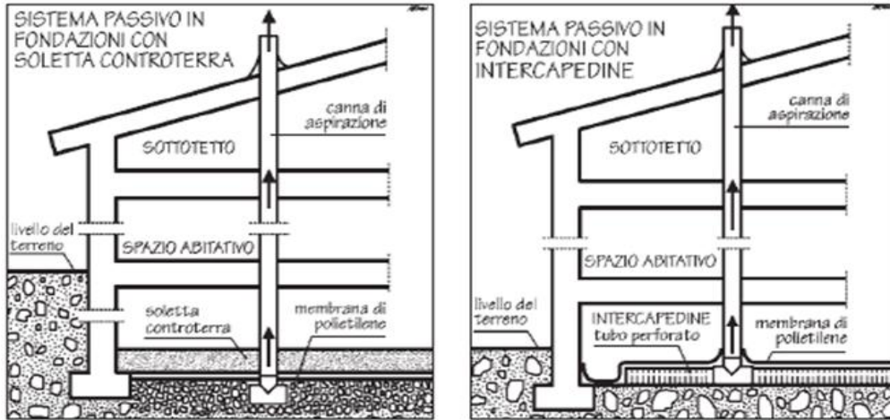
Fig.1 – Sistema passivo in fondazioni con soletta controterra; Fig 2 – Sistema passivo in fondazione con intercapedine.
