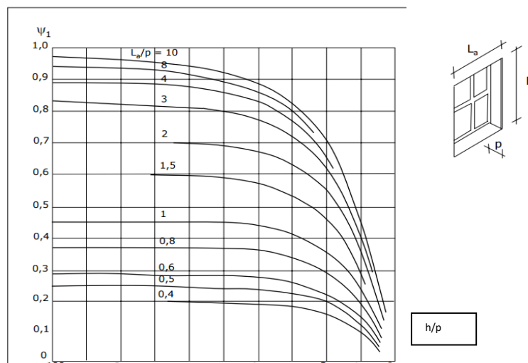
Grafico D.1.4.c – Fattore di riduzione apertura verticale \Psi_1
